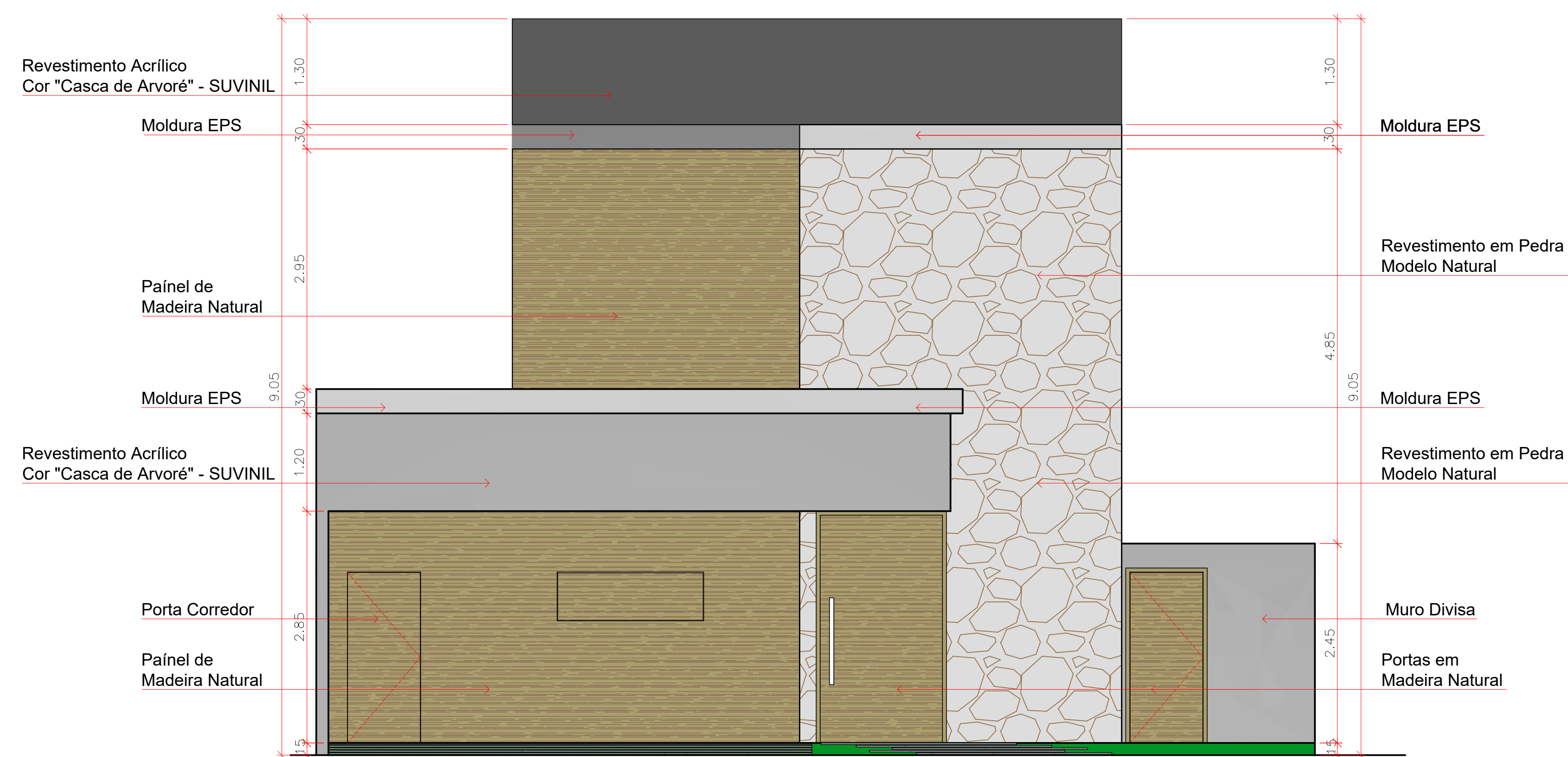
Fachada Frontal
