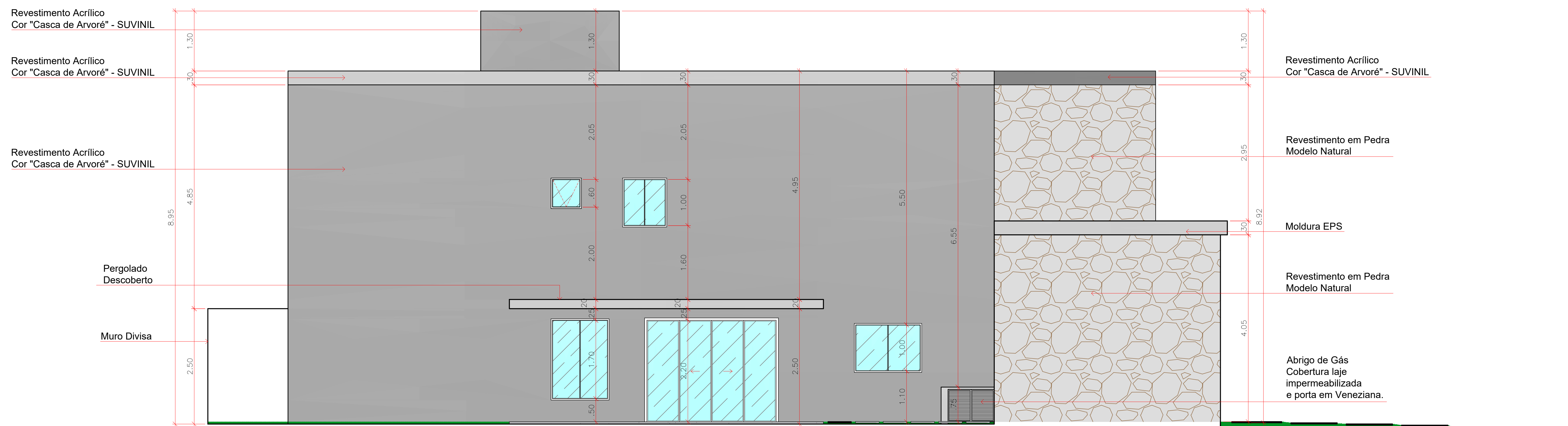
Fachada Lateral Esq.
