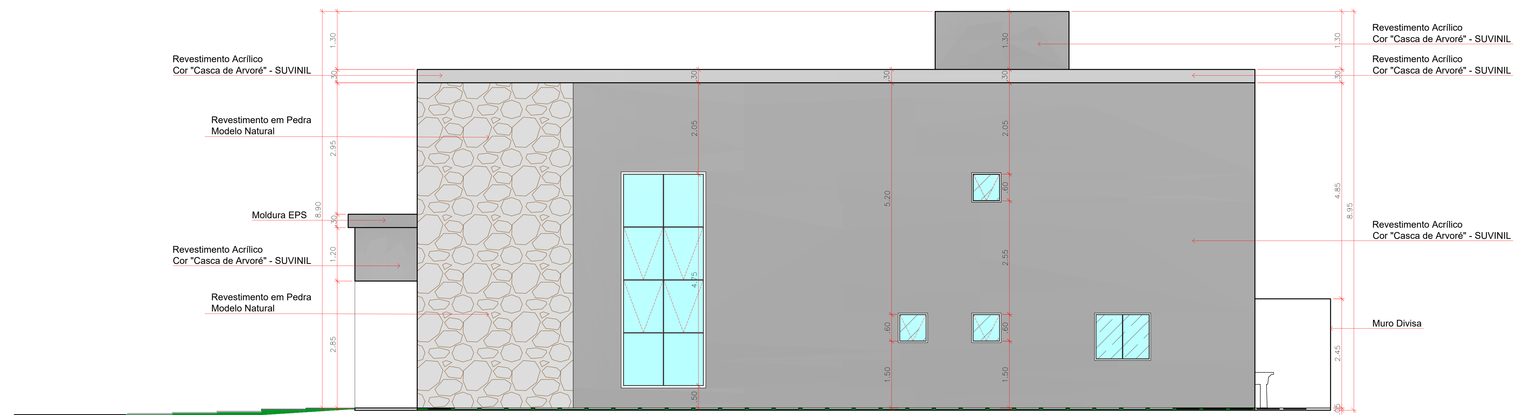
Fachada Lateral Dir.
