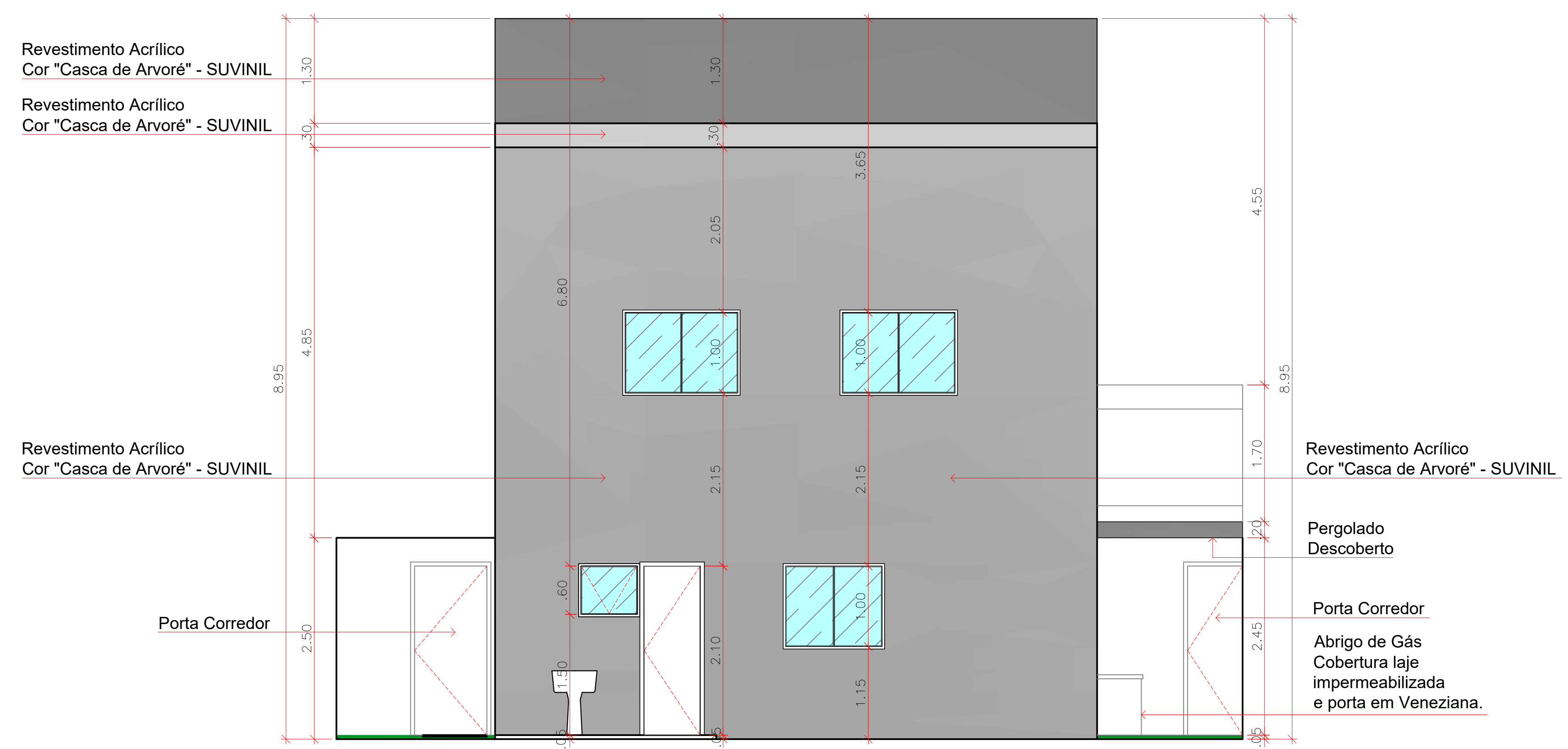
Fachada Fundos
